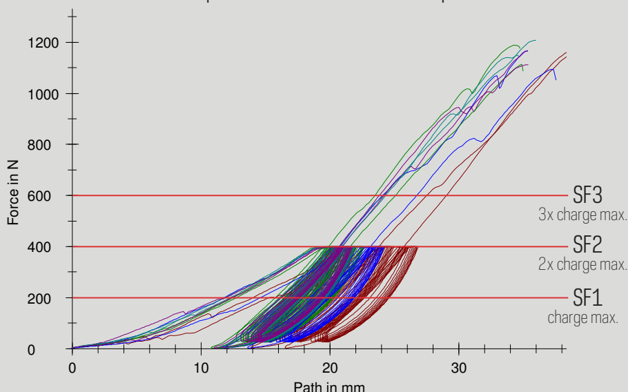
exemple de résultats d'essai Micro Grip
