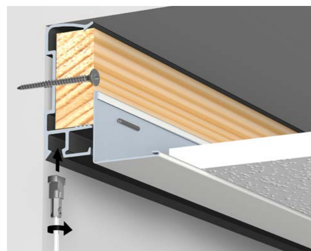
ART STRIP (ICM SYSTEEMPLAFOND)
